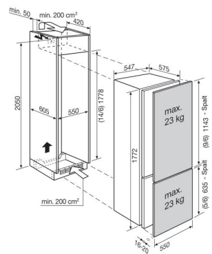
IK307BN / IK305BN Möbelfronten auf Gerätetüren verschraubt
