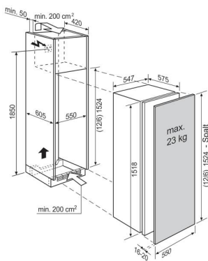
IK285SA / IK283SA Möbelfronten auf Gerätetüren verschraubt
